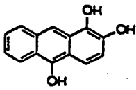
ANTHRAROBIN
